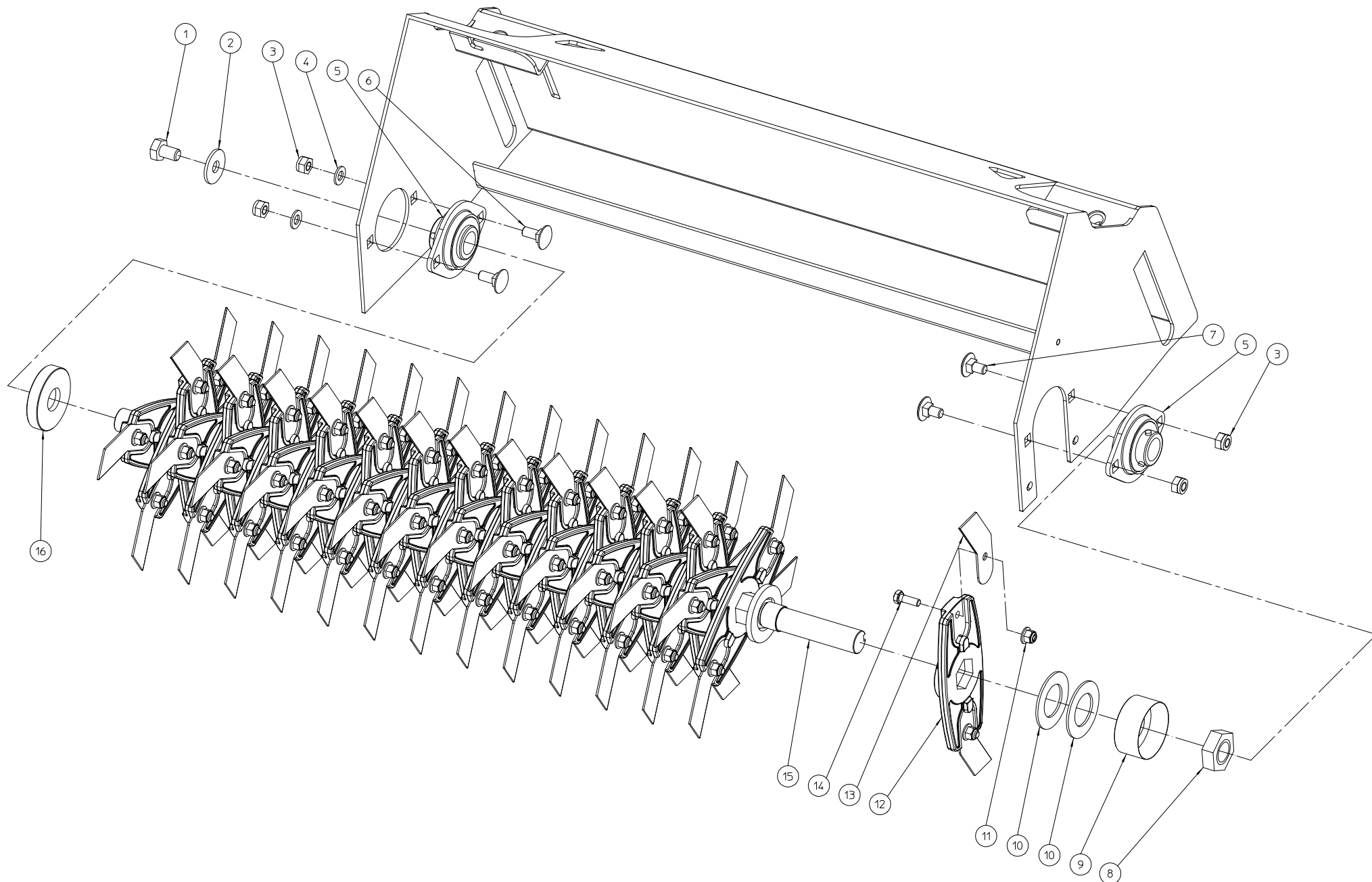
ELIET E650ZR -- BLADE SHAFT
